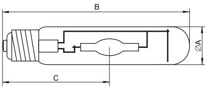
Рисунок 3. Лампа металлогалогенная с трубчатой колбой цоколь E40.
